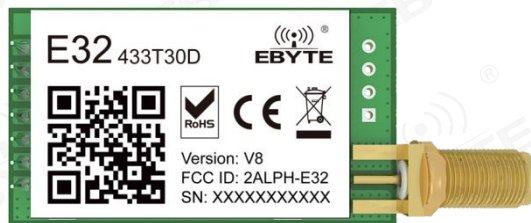
图 2: E32-433T30D
