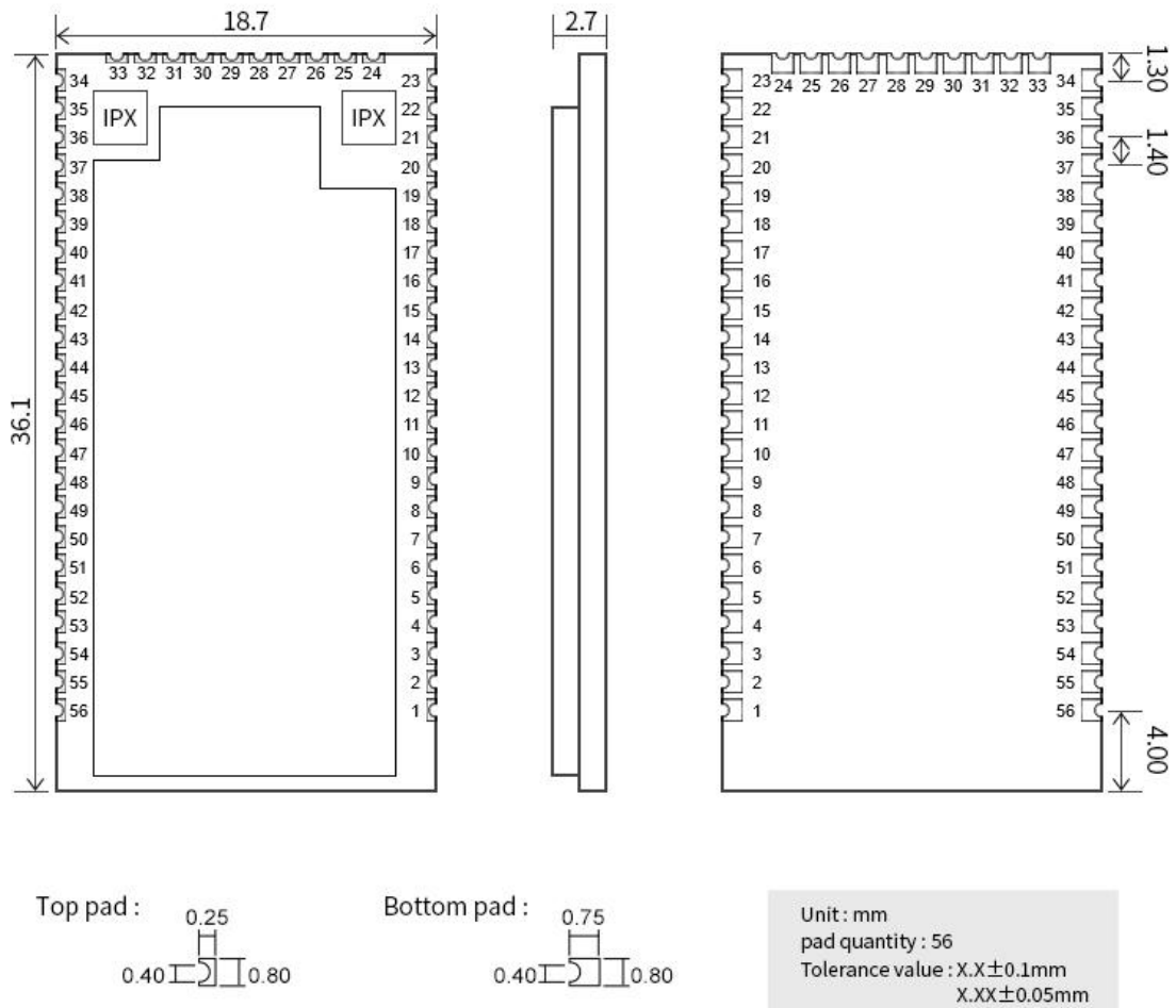
图 2: E103-W20(7628)尺寸图
