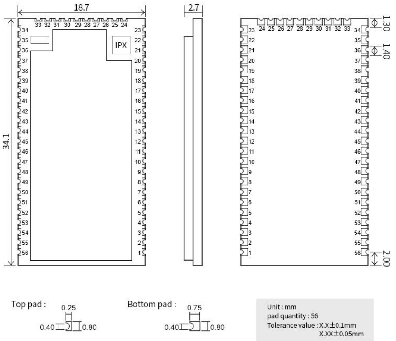
图 1: E103-W20 (7688) 尺寸图
